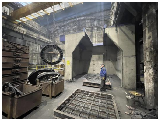
F3, odprašení velkého vytloukacího roštu.
