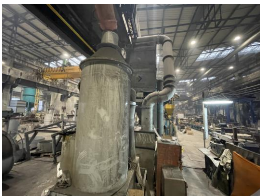
Jaderna, záchyt TZL a neutralizace DMEA, dřívější instalace.
